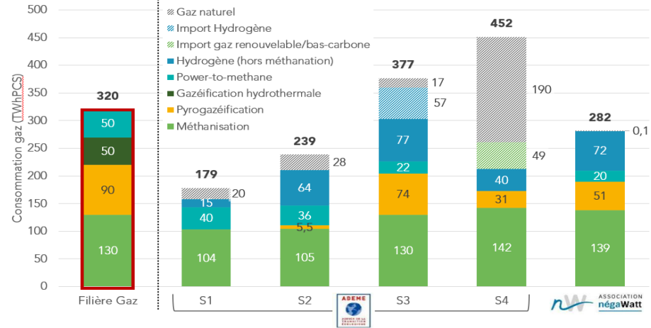
SCÉNARIOS DU MIX GAZIER EN FRANCE À HORIZON 2050 (TWh PCS)
